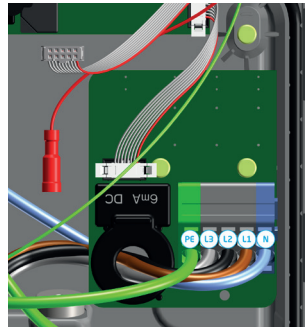
Figuur 8b: Aansluitklemmen voeding en Control Pilot (CP) connector voor laadkabel (rood) bij S-line 3-fase en Pro-line
