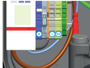
Figuur 8a: Aansluitklemmen voeding en Control Pilot (CP) connector voor laadkabel (rood) bij S-line 1-fase
