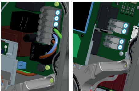
Figuur 7a en 7b: Aansluitpunten voor aders van de laadkabel S-line 1-fase (links) en S-line 3-fase en Pro-line (rechts).
